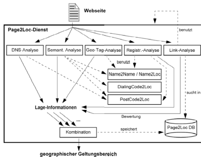
Abb. 3: Integration der Link-Analyse in den „Page2Loc“-Dienst.
